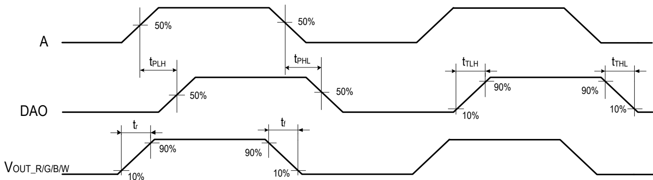
Fig. SM18522P 动态参数测试示意图
