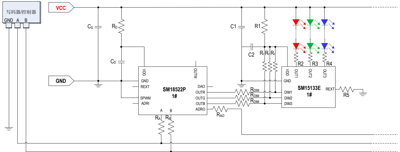
Fig. SM18522P+SM15133E 组合应用方案图
