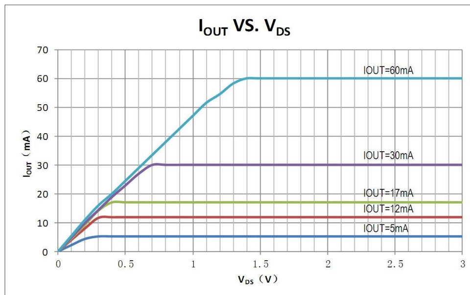
Fig. SM18522P 输出电流 I_{OUT} 与 OUT 端口电压 V_{DS} 的关系图
