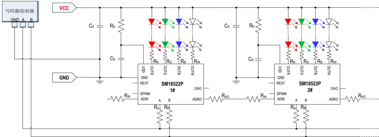
Fig. SM18522P 典型应用方案图
