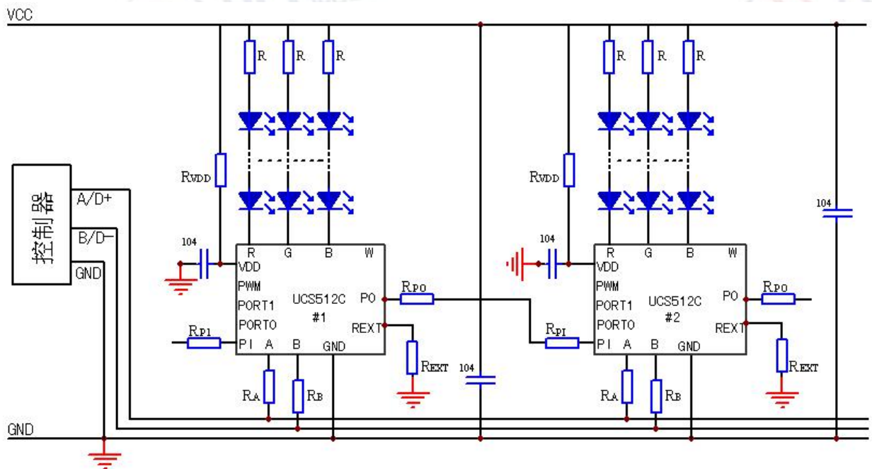
应用图 2：RGB 3 色应用
